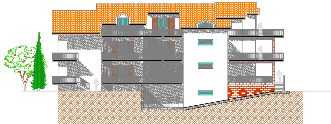
PROSPETTO SUD rapp. 1:100
